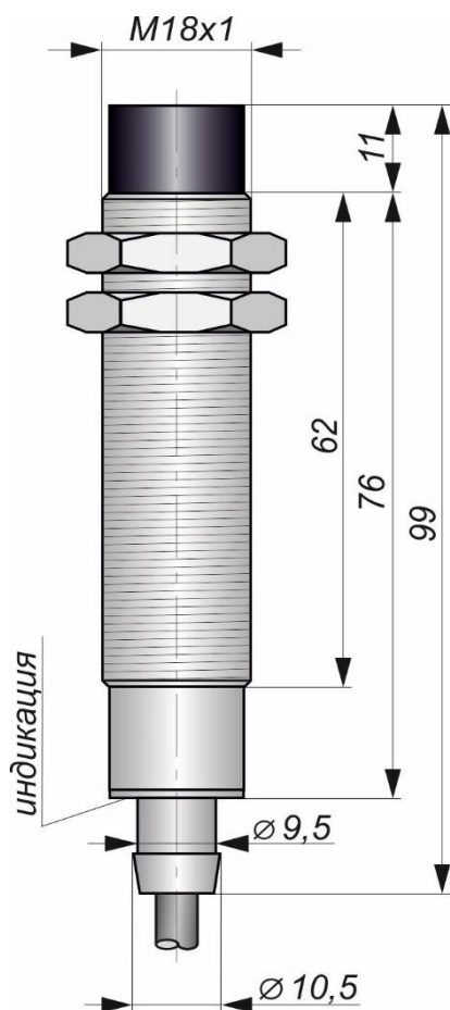
Габаритный чертеж
